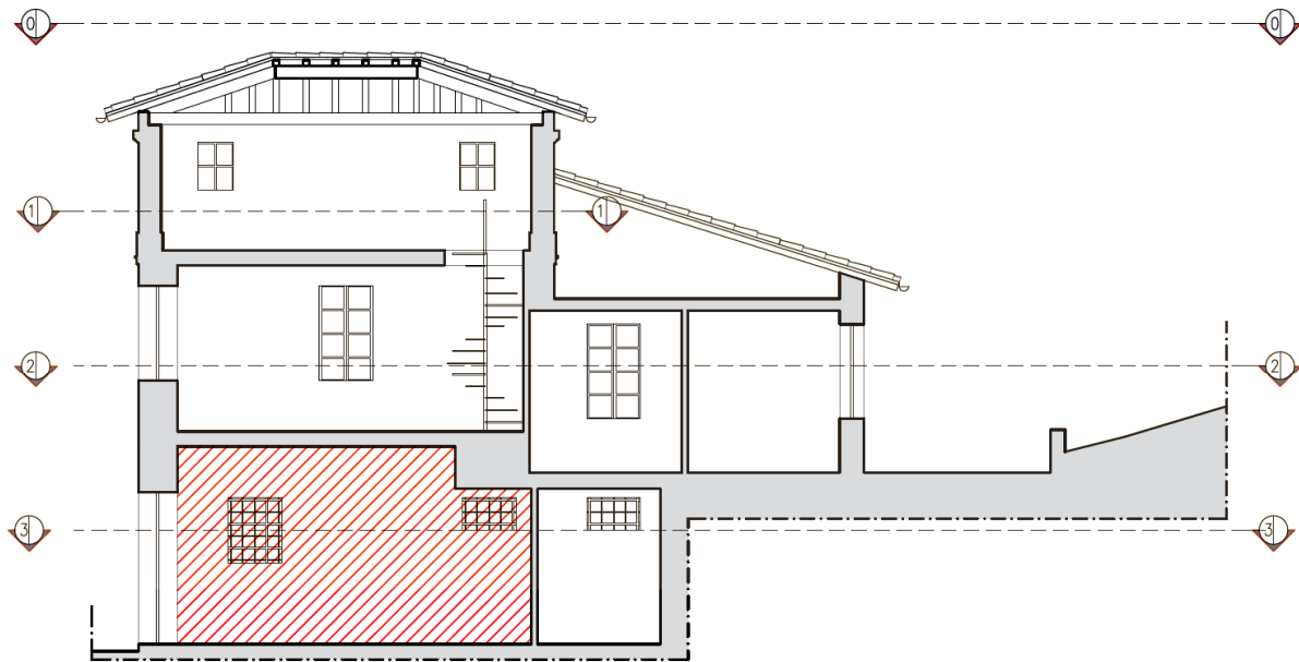
SEZIONE B-B
