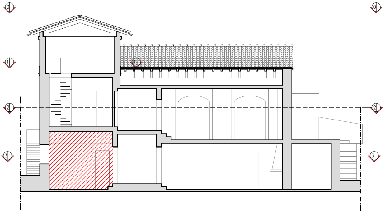
SEZIONE A-A
