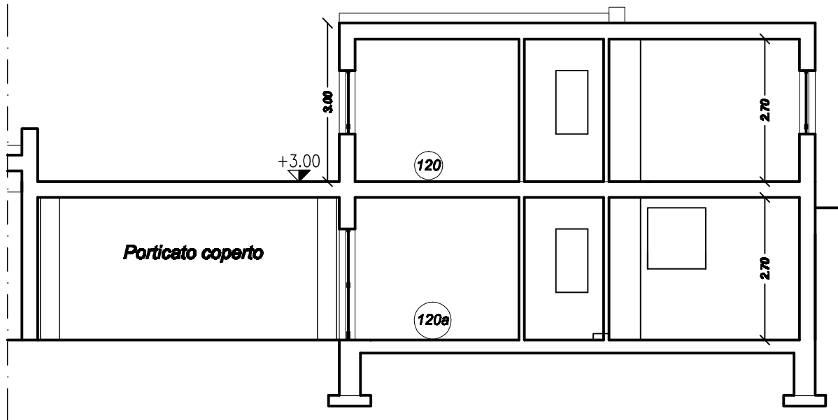
Sezione A-A'
